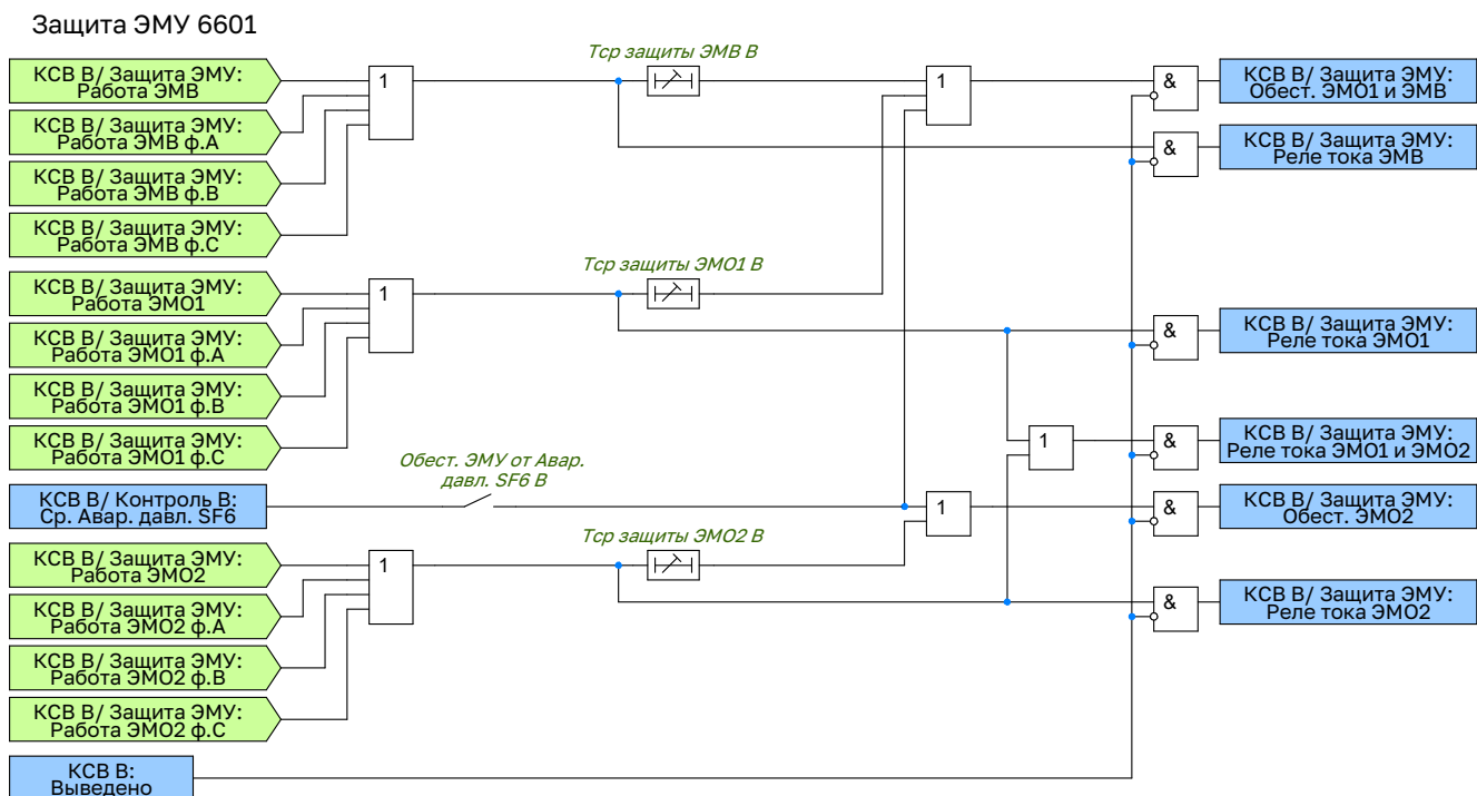
Рисунок 2.33 – Функциональная схема логики защиты ЭМУ выключателя
