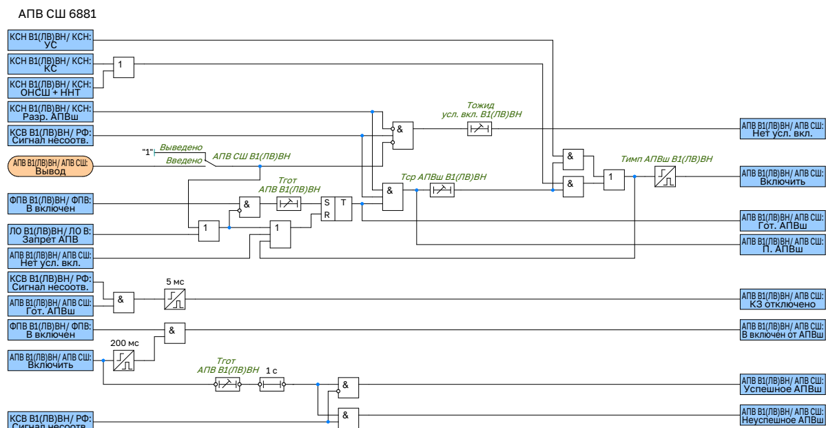
Рисунок 2.30 – Функциональная схема логики АПВ СШ В1(ЛВ) ВН
